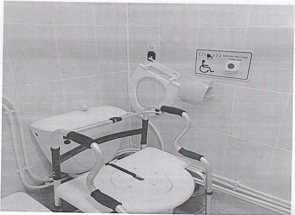
Установка унитаза с функцией подогрева воды и сиденьем-биде. Установка поручней и кнопки вызова помощи.
